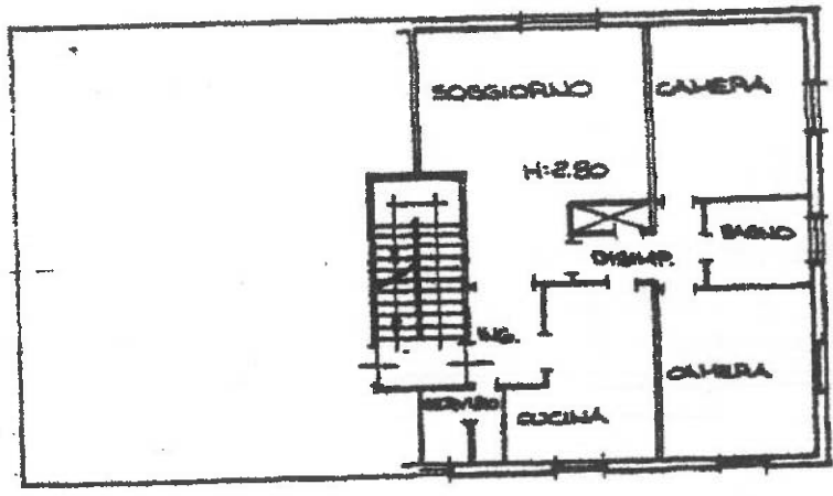
PIANO SECONDO
